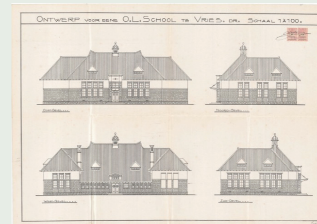
Bestektekeningen 'Ontwerp voor eene O.L. School te Vries' (1915)
